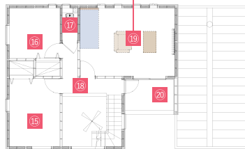
▲ 2F 平面図
